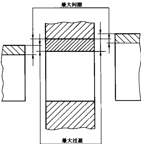
图 5 过渡配合
