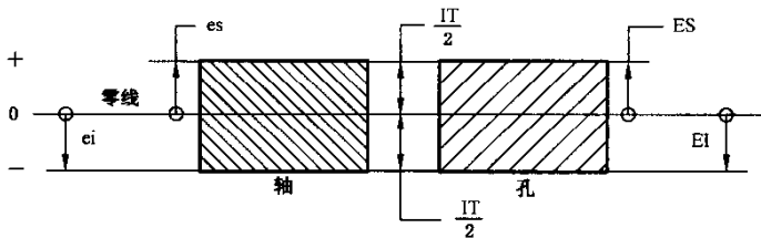
图 19 偏差 js 和 JS
