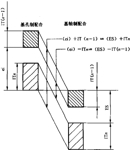
图 A.1 A.3.2b) 中给定规则的图解
