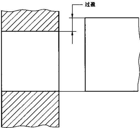
图 6 过盈
