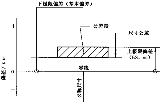
图 2 公差带图解
