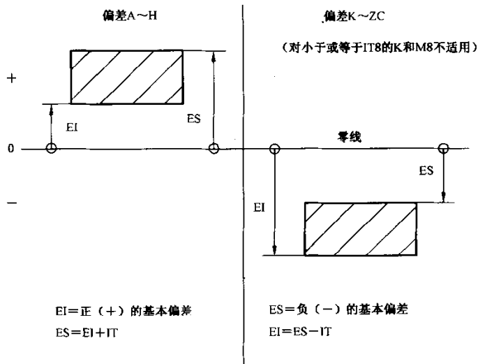
图 18 孔的偏差
