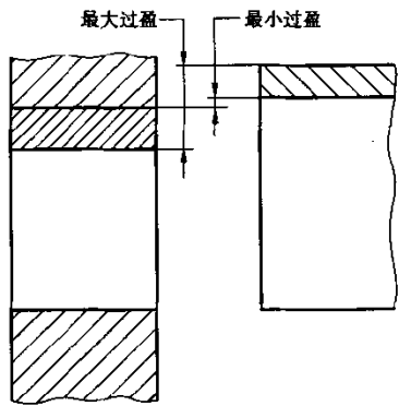
图 7 过盈配合
