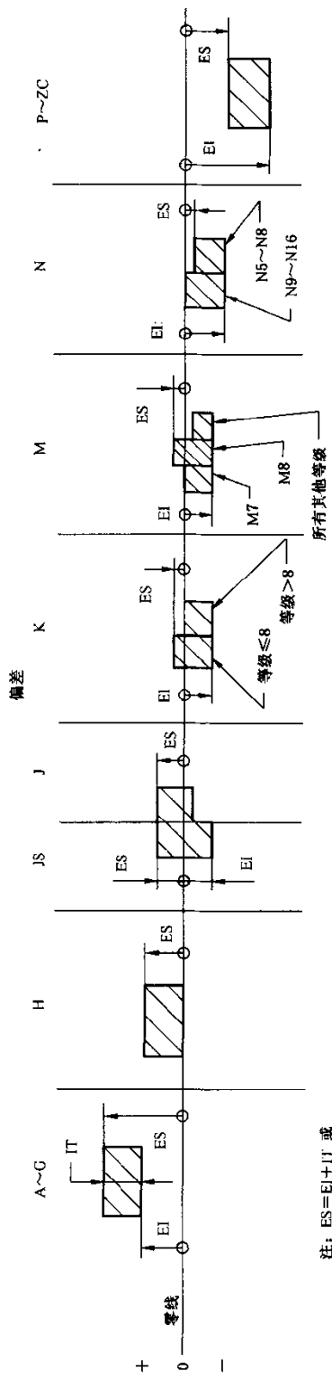
a) 孔
