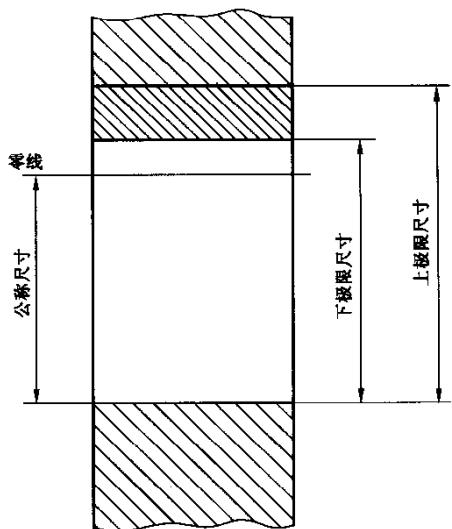
图 1 公称尺寸、上极限尺寸和下极限尺寸
