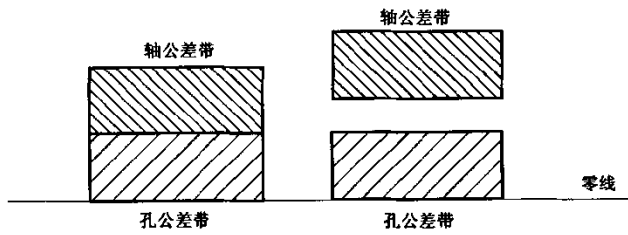
图 9 过盈配合的示意图
