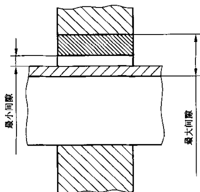
图 4 间隙配合
