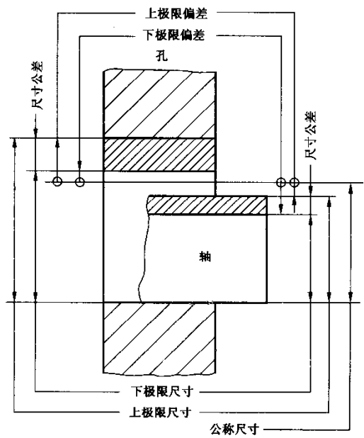
图 15 术语图解
